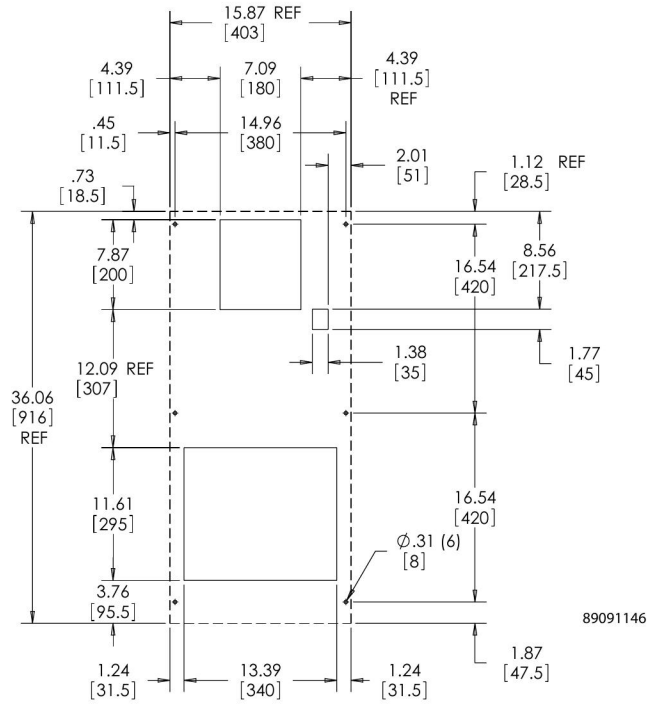
CUTOUT DIMENSIONS
